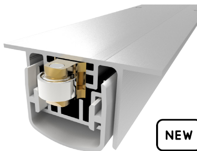
DS-298XL298RP Rolling push button in brass with inox ball bearing Pulsante di spinta rotante in ottone con cuscinetto inox
