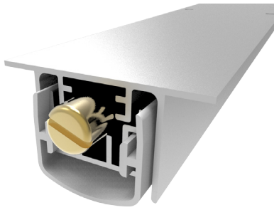
DS-298XL298RT Round push button in brass Pulsante di spinta tondo in ottone
